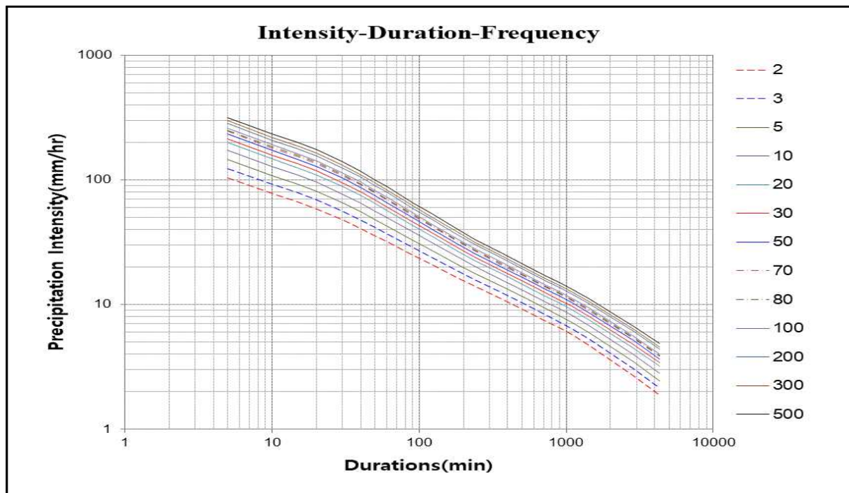
【그림 42.9】 영천지역 IDF곡선
