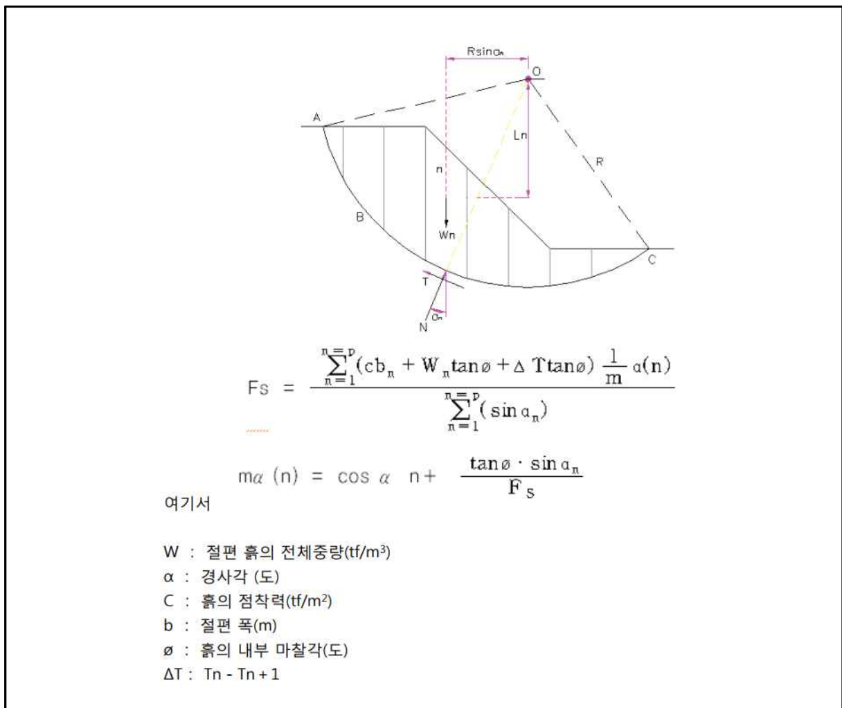
【그림 42.7】 Bishop의 안전율 계산식
