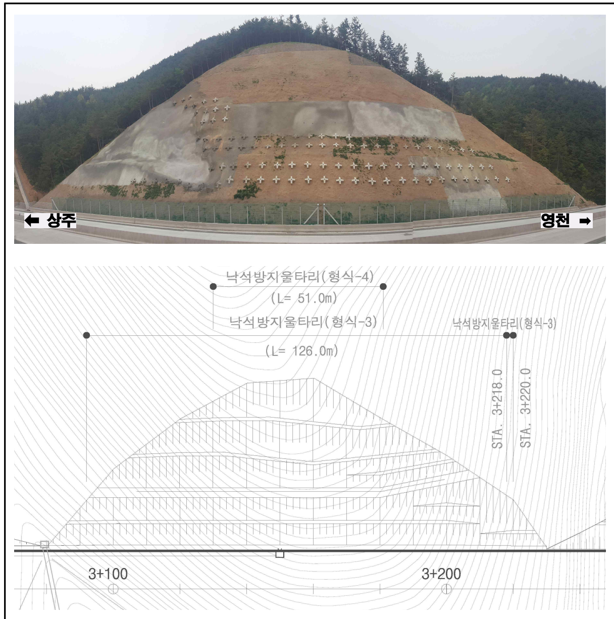
【그림 42.14】 상주절토42 검토대상 비탈면구간
